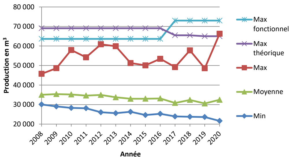
Figure 2.3 Évolution de la production journalière annuelle de l'usine 2008-2020
